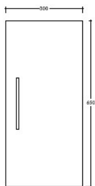
Vista frontale
